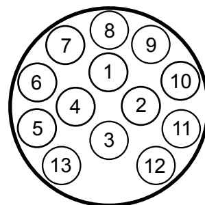
DIN/ISO 11446 13-pol
